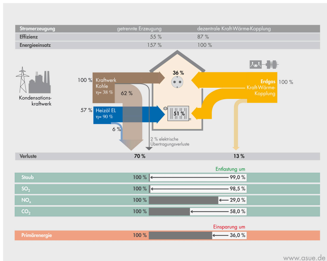
Abbildung 5.4: Vergleich der Effizienz und Umwelteigenschaften von Kohle- mit Blockheizkraftwerken (Quelle: asue.de [3])
