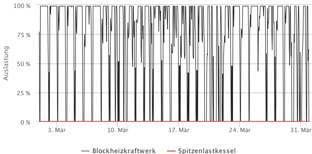
Abbildung 5.9: Nicht optimierte Fahrweisen von BHKW und SLK
