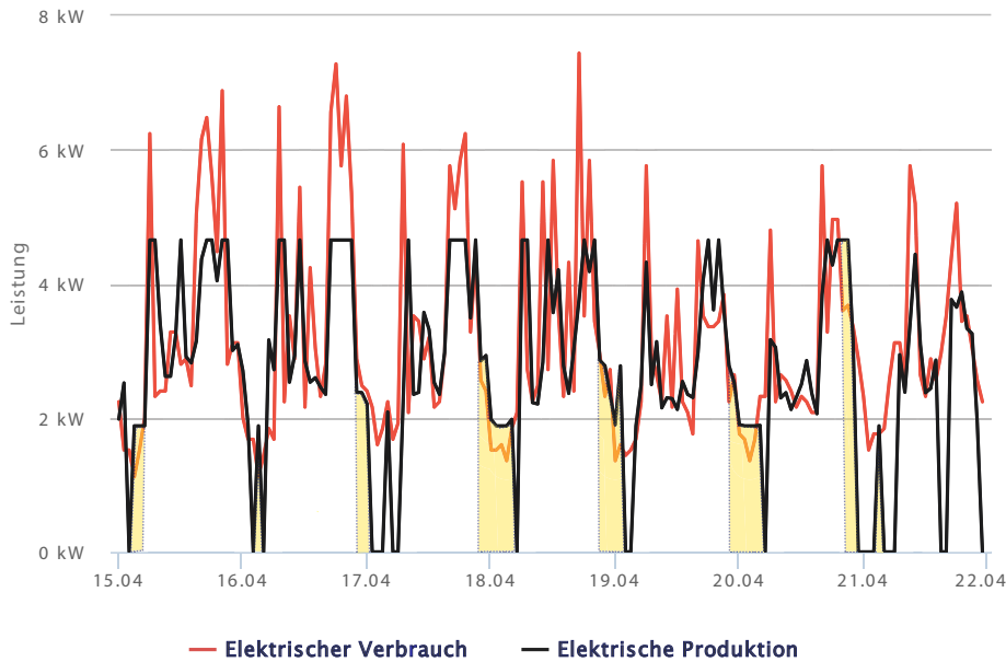
Abbildung 4.11: Stromproduktion mit Maximierung des Eigenverbrauchs (in gelb)
