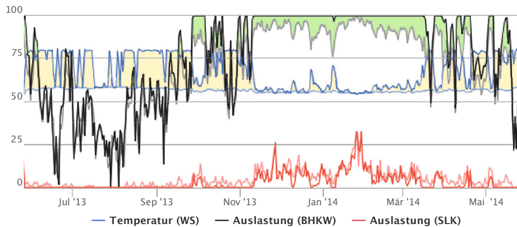
Abbildung 5.8: Vorhersagen-basierte Optimierung von BHKW und SLK; die wichtigen Bereiche wurden eingefärbt
