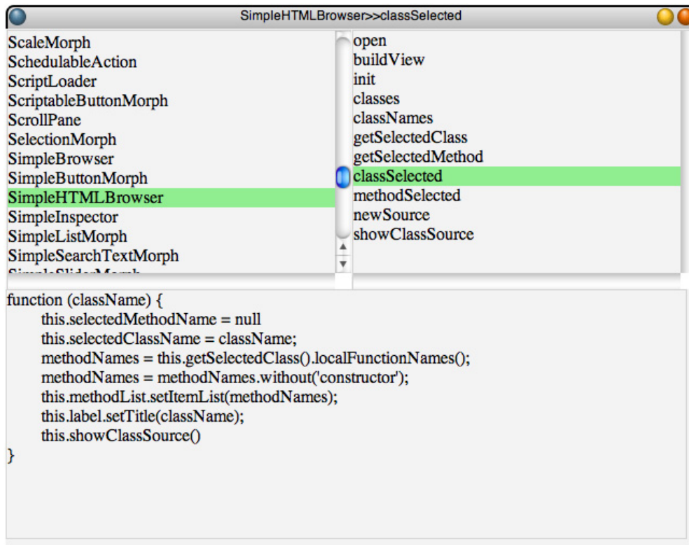
Fig. 5: HTML browser.
