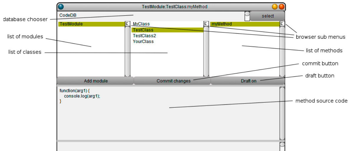
Fig. 4: The Code Database Browser
